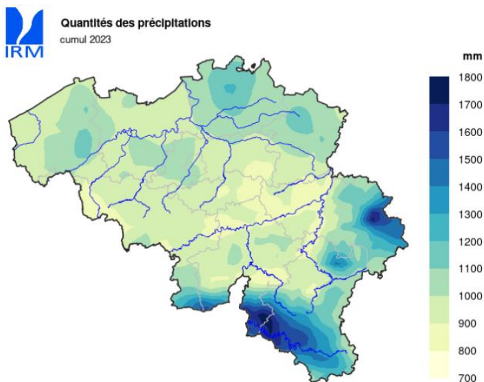
Ilustración 2 Precipitaciones acumuladas 2023. Fuente: Institut Royal Météorologique. Bilan climatique annuel. Année 2023.
