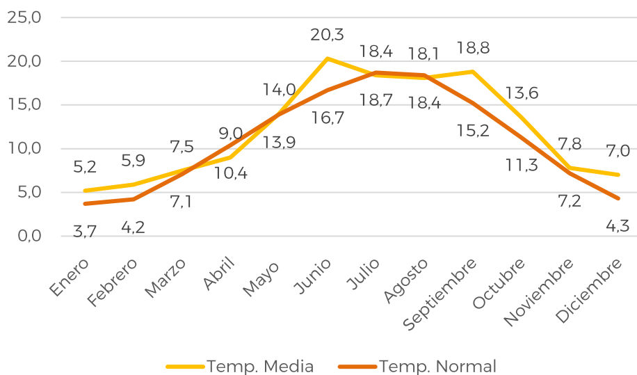
Valor de las temperaturas medias mensuales 2023
